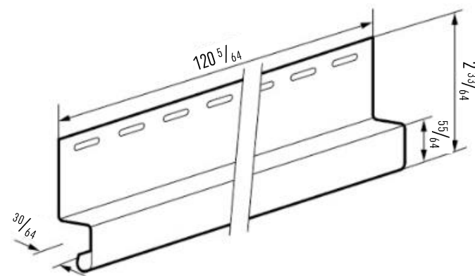
SV(P) 16.5 Drip edge
