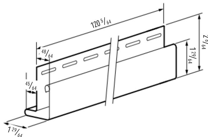
SV(P) 12.5 Outside corner mini
